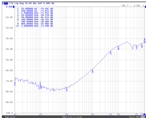
PSRR
